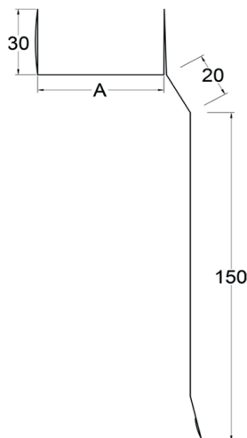
CANAL U CON BOTA AGUA MEDIDA VARIABLE
