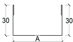
CANAL U TÍPICO
